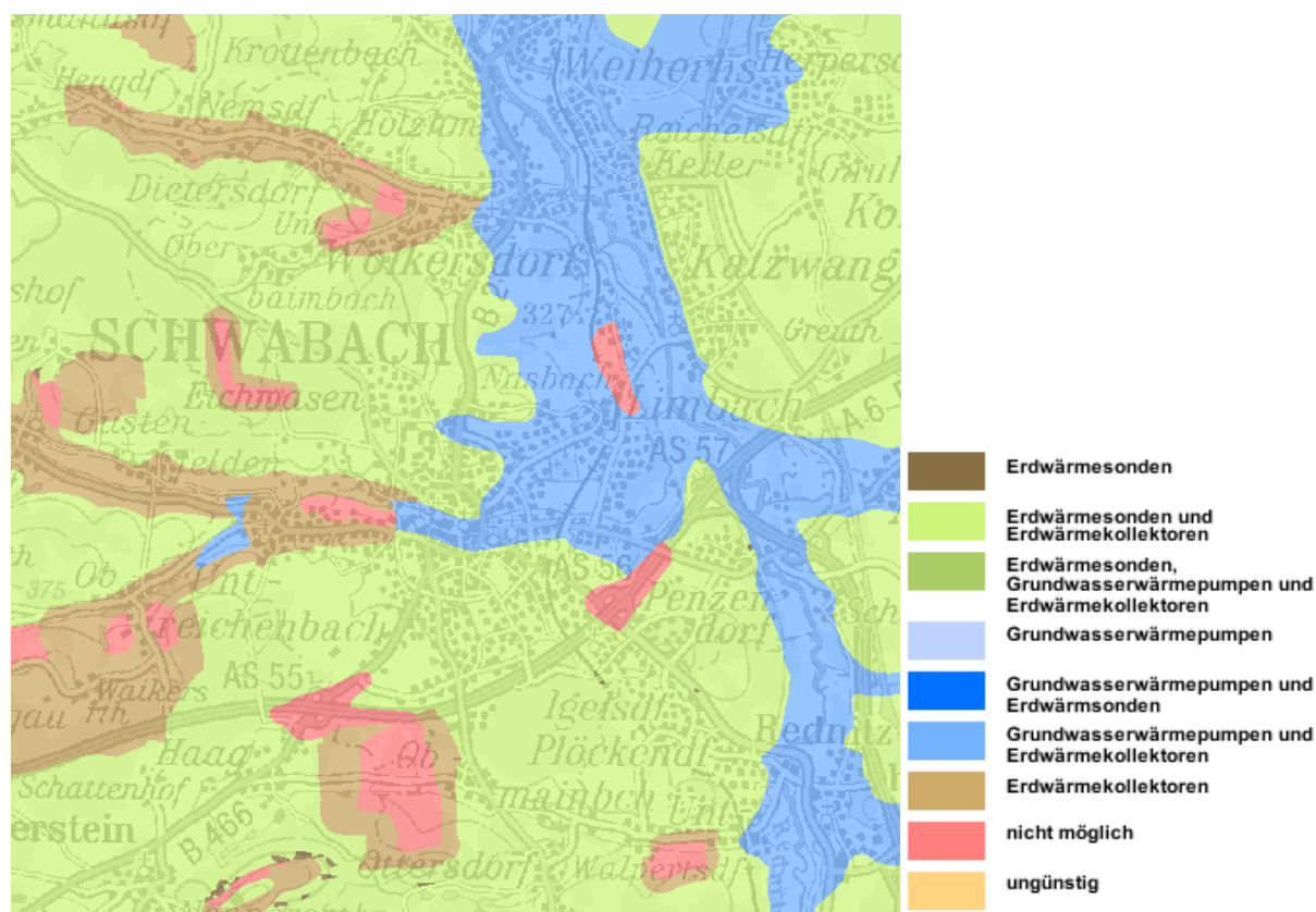
Abbildung 9: Für oberflächennahe Geothermie geeignete Gebiete in Schwabach
