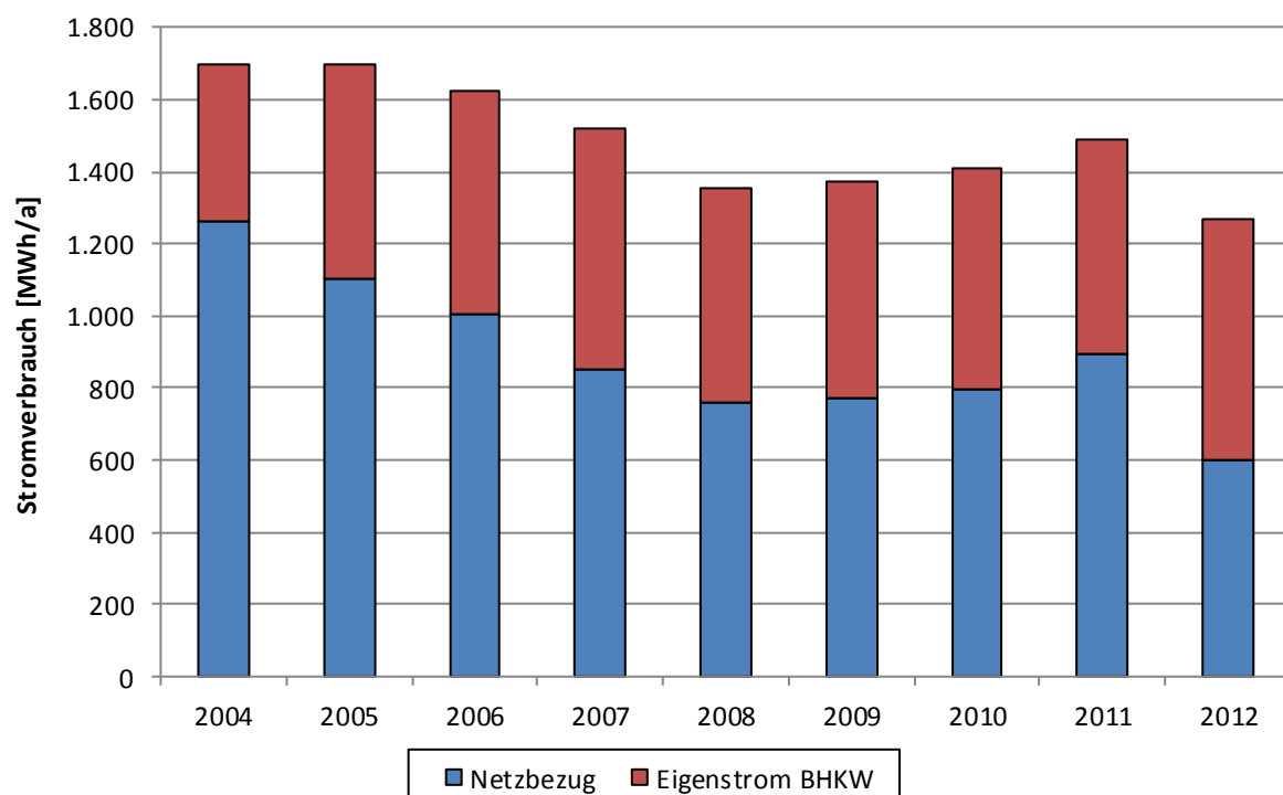
Abbildung 6: Der Stromverbrauch der Kläranlage Schwabach
