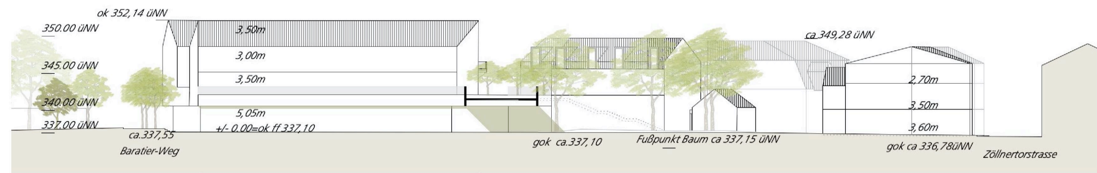
ansicht südfassade
